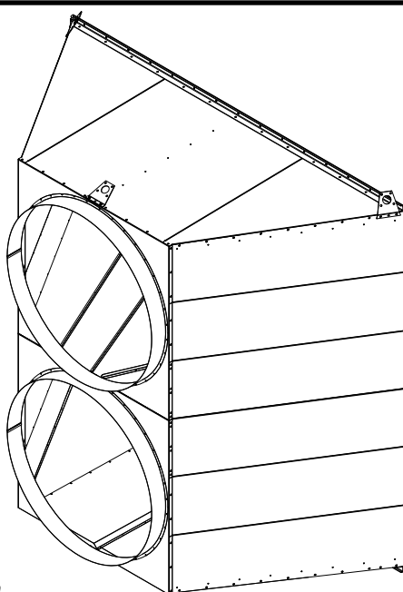
A75038 koonus kokkupanduna
