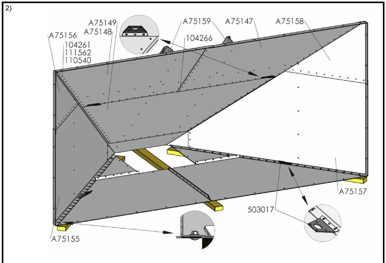
Kuva 2): Lukkokantaruuvien kanta ulospäin (betonia vasten). Asennetaan nostokorvat (4 kpl). Pitkien reikien liitokset jätetään löysälle (säätövara).
