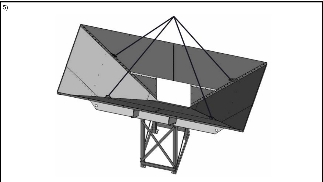
5. attēls.: Piltuves uzstādīšanai bedrē nepieciešams pietiekami spēcīgs celšanas aprīkojums. Celšanai izmantojiet četras ķēdes.
