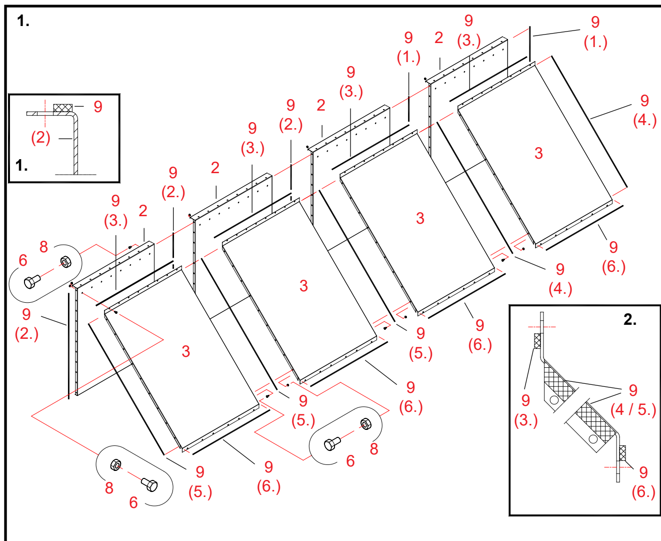
Asamblarea capătului canalului de aer A70748 – continuare
