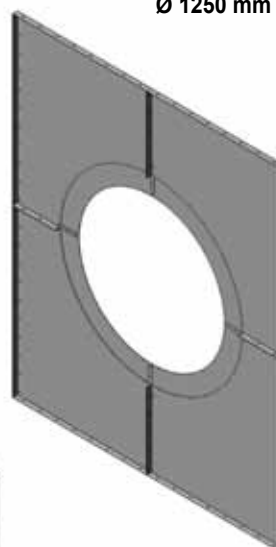
A71245 – gură laterală Ø 1250 mm / Ø 1000 mm
