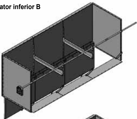
A70824 - obturator de canal B
