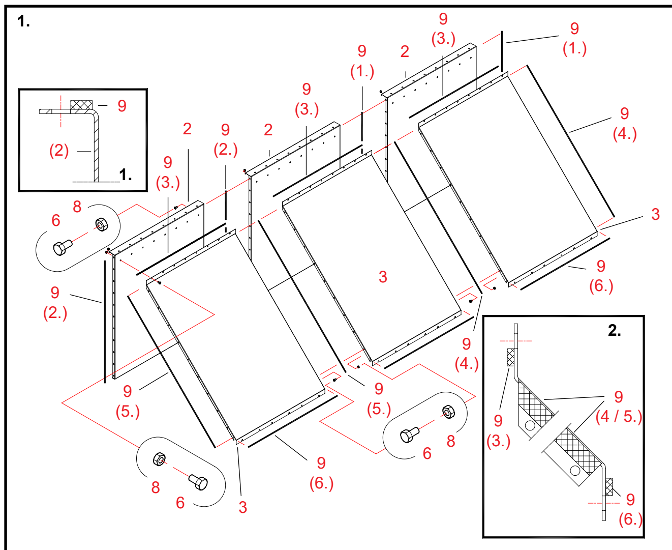
Asamblarea capătului canalului de aer A71013, continuare
