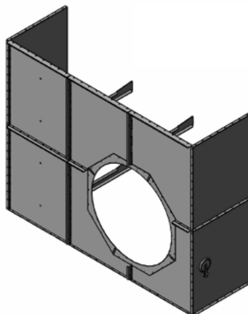
A71403 – piesă centrală S Octogonal / Ø 1250 mm
