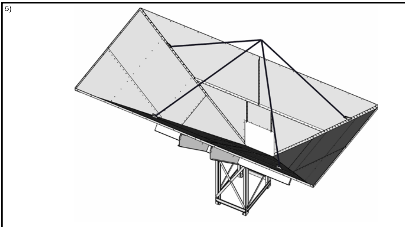
5. attēls.: Piltuves uzstādīšanai bedrē nepieciešams pietiekami spēcīgs celšanas aprīkojums. Celšanai izmantojiet četras ķēdes.
