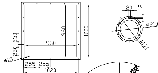
Tuhkaruuvien laippojen ulkomitta
