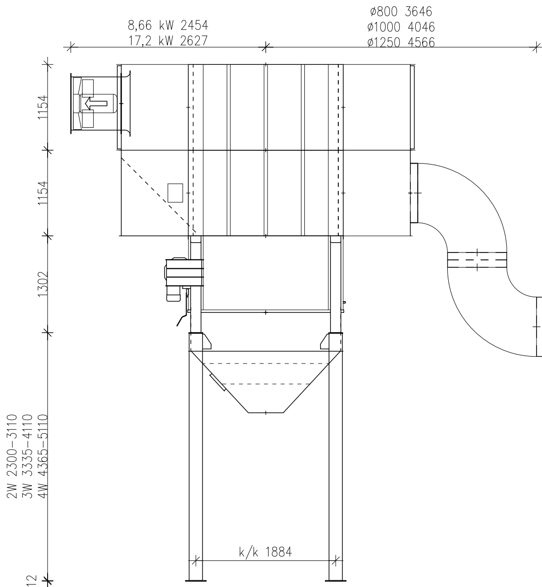
ILMAPÄÄDYT 1,0 M / AIR CHANNEL 1,0 M
