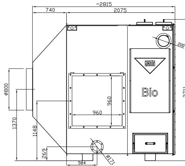
Tuhkaruuvien laippojen ulkomitta
